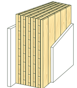
Außenwand – 11 Lagen mit Innenbeplankung und dünner Außendämmung
