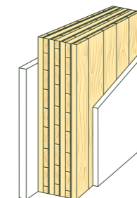
Innenwand – 7 Lagen mit beidseitiger Innenbeplankung
